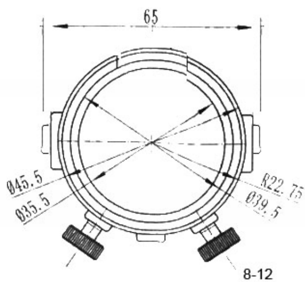
Korpus prowadnicy
